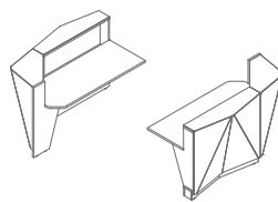
ALP18L 1806 / 946 / 1100 90 kg
