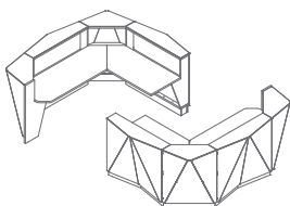
ALP19L 2514 / 1907 / 1100 172,5 kg
