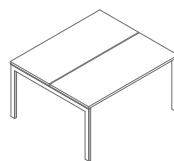
BOU54 1400 / 1210 / 740 54 kg
