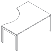
BOU25 1800 / 1200 / 740 51.2 kg
