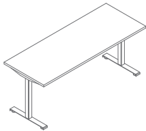
BOT587 1800 / 700 / 740 46.85 kg
