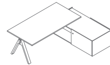
V06P 2000 / 1000 / 740 194.94 kg
