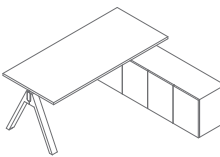
V204P 2000 / 1700 / 740 137.6 kg
