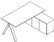
V163P 1600 / 1300 / 740 112.5 kg
