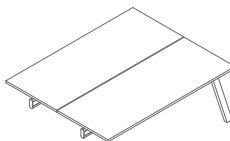
V220L 2000 / 1610 / 740 170.2 kg
