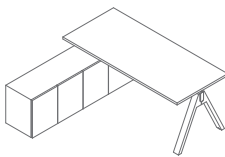
V184L 1800 / 1700 / 740 130.55 kg
