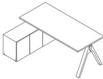
V183L 1800 / 1300 / 740 119.55 kg
