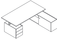
V10P 2000 / 1800 / 740 203.44 kg
