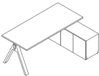
V183P 1800 / 1300 / 740 119.55 kg
